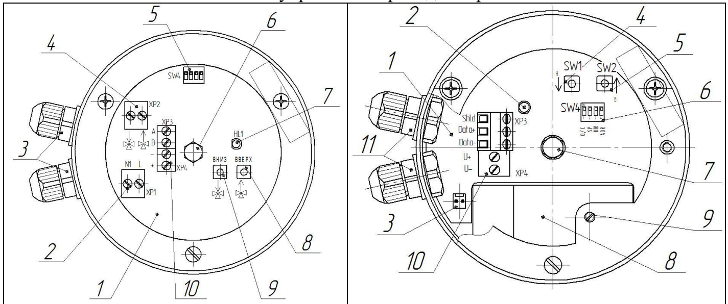
Рисунок Е.1 – Привод ЭП-100 и ЭП-180 с открытой крышкой
