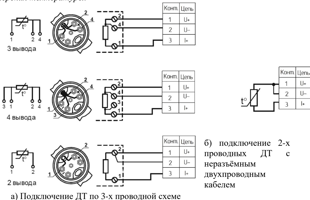
Рисунок 23 – Подключение ДТ
