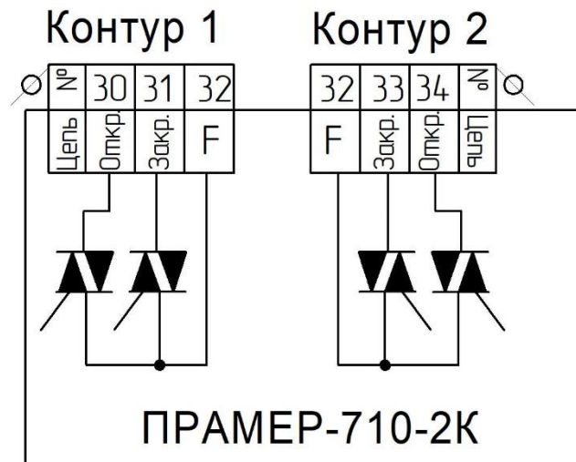
Рисунок 24 – Подключение ИМ
