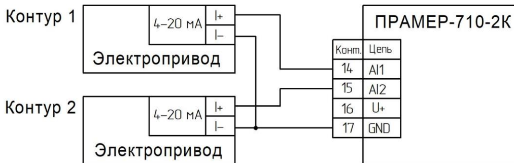
Рисунок 29 – Подключение датчика положения привода ИМ.
